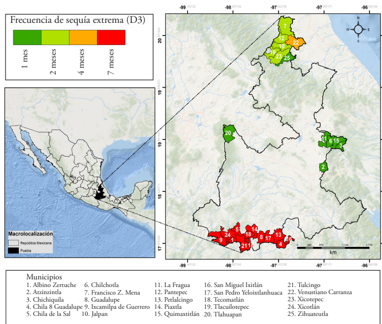
Fuente: elaboración propia con datos del Monitor de Sequía de México [MSM] (2023). Figura 2. Ubicación de municipios con reporte de sequía categoría extrema y su frecuencia en meses.
