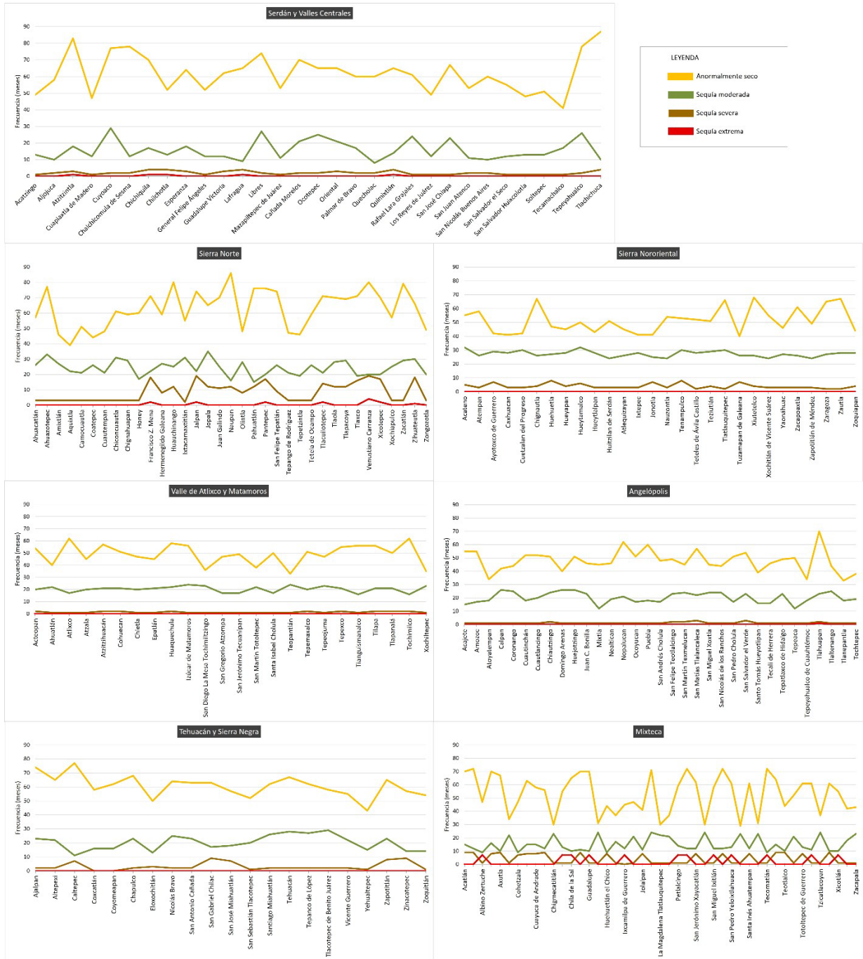
Fuente: elaboración propia con datos del Monitor de Sequía de México [MSM], (2023). Figura 3. Frecuencia de eventos de sequía en Puebla por región y municipio de 2003 a 2022.
