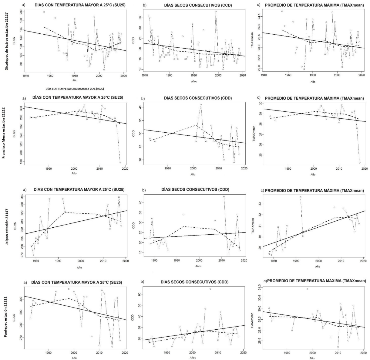
Figura 4. Resultados del tratamiento de bases de datos de estaciones meteorológicas con RClmDex.
